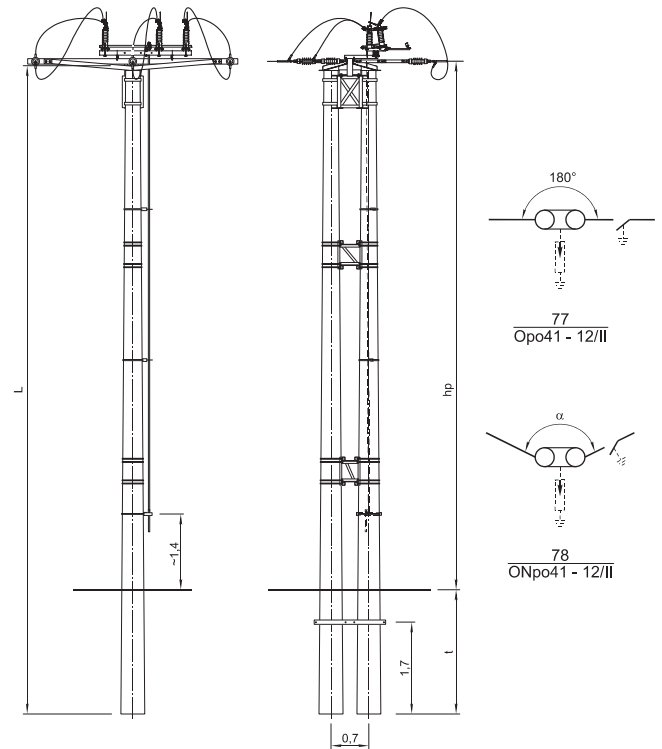
SŁUPA ODPOROWY Opo41 i ODPOROWO-NAROŻNY ONpo41÷ONpo43 Z ODŁĄCZNIKIEM ON M III SA, OUN M III SA LUB ROZŁĄCZNIKIEM RN M III SA, RUN M III SA WARIANT I
