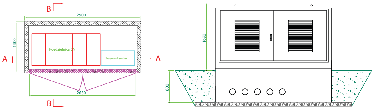
Front złącza
