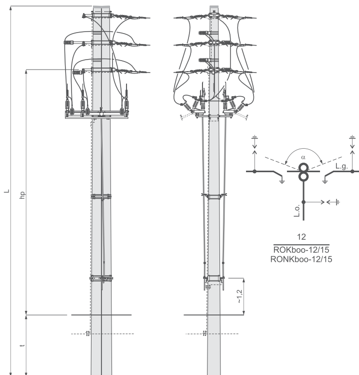
Słup rozgałęźny odporowo - krańcowy bliźniaczy ROKboo-□/□ i rozg. odp. - narożno krańcowy bliźniaczy RONKboo-□/□ z rozłącznikiem FL□GBW-I lub FL□GBWu-I i rozłącznikiem FL□GBWL-I lub FL□GBWLu-I
