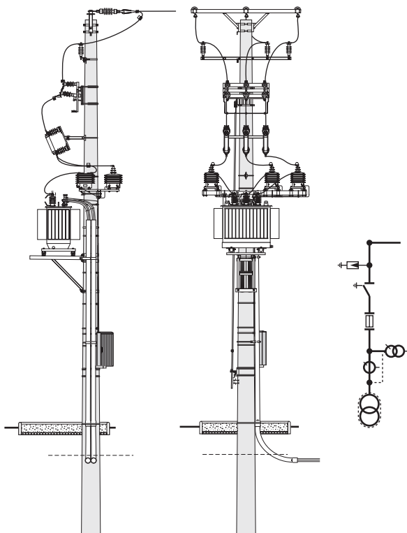
STSRS - 20/630-I-□/□- 2 - OP3
