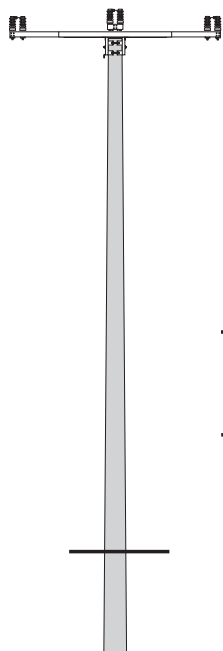
Słup przelotowo - skrzyżowaniowy PS1 - □/10□ i narożno - skrzyżowaniowy NS1-□/□□
