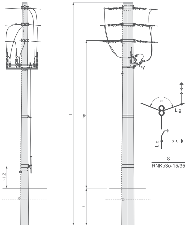
Słup rozgałęźny narożno - krańcowy bliźniaczy RNB3o-□/□ z rozłącznikiem FL□GBW-I lub FL□GBWu-I
