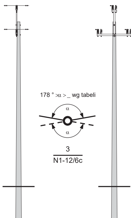
Słup przelotowy P1 - □/□□ P2 - □/ ŻN □
