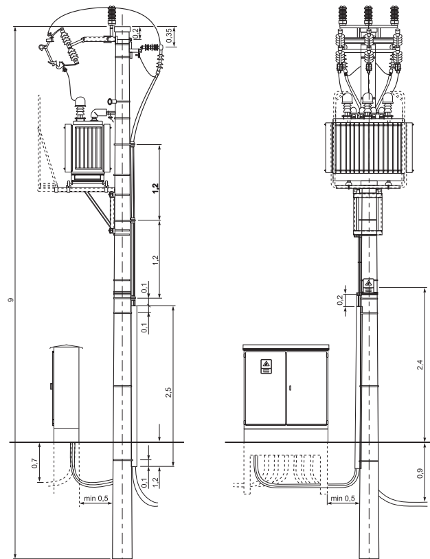
STSR - 20/400 - KK2
