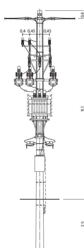
STNK-20/□/1/PP3, STNK-20/□/3/PP3
