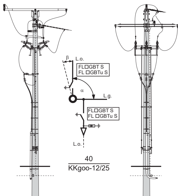
Słup podporowy KKgoo - □/□ z głowicami kablowymi i dwoma rozłącznikami FLGBT S lub FLGBTu S
