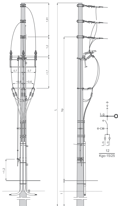
Słup krańcowy Kgo - □/□□ z dwoma kompletami głowic kablowych i rozłącznikiem FL□GBT S lub FL□GBTu S
