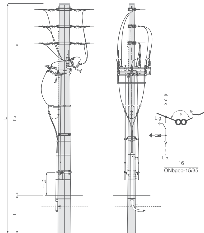
Słup odporowo-narożny ONbgoo-□/□ bliźniaczy z głowicami kablowymi i rozłącz. FL□GBT S lub FL□GBTu S oraz rozłącz. FL□GB□-I lub FL□GB□u-I
