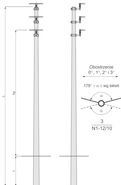
Słup narożny N1 - □/□□ \alpha \geq 150^\circ
