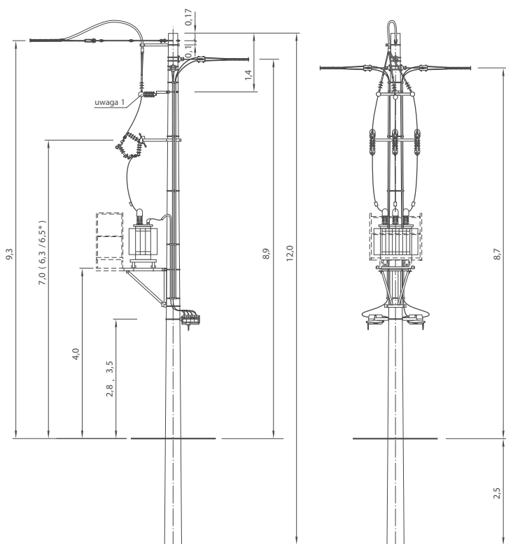
STNKs-20/□/I, STNKp-20/□/I
