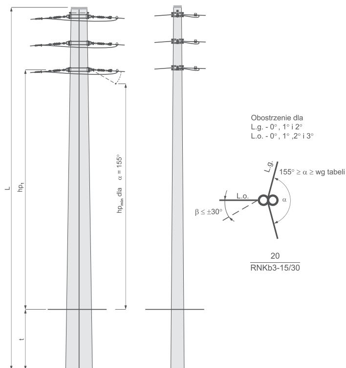
Słup rozgałęźny narożno - krańcowy bliźniaczy RNKb3 - □/□
