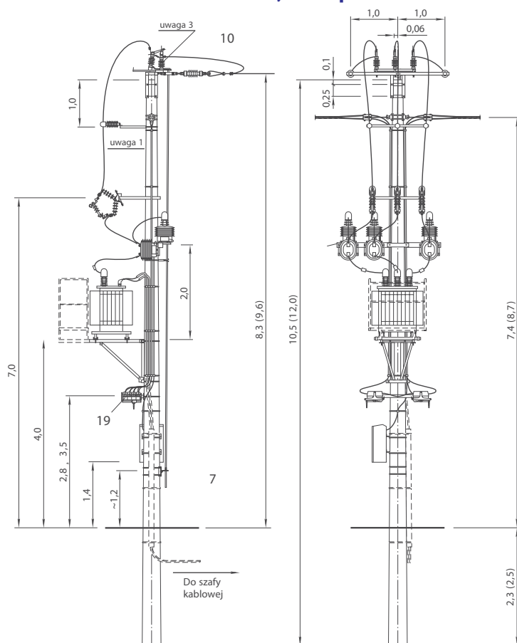
STNo-20/□/PP3
