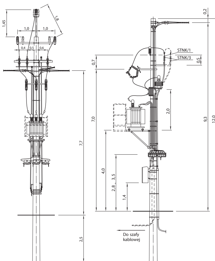
STNK-20/□/1/PP3, STNK-20/□/3/PP3
