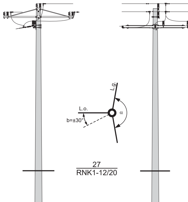
Słup rozgałęźny narożno - krańcowy RNK1 - □/□
