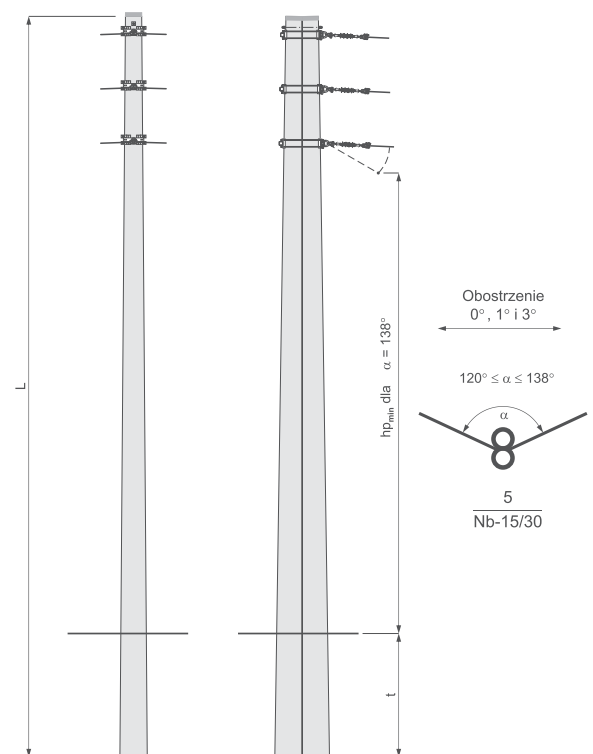
Słup narożny bliźniaczy Nb - □/□
