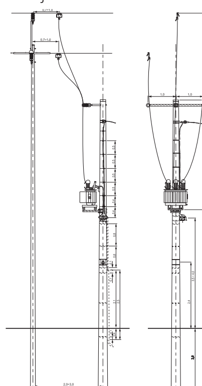
STSR - PO - 20/25/3 - w/2
