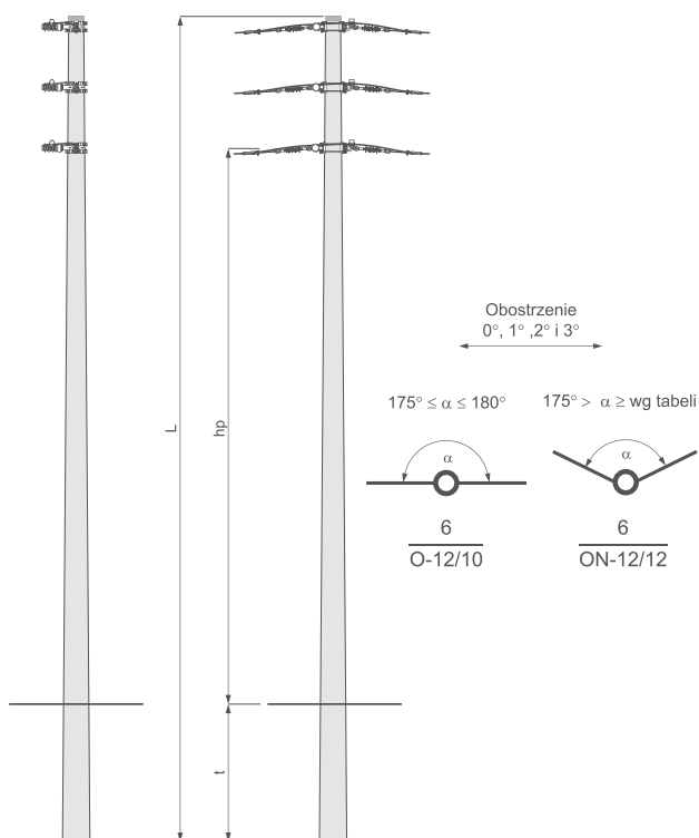
Słup odporowy O - □/□□ i odporowo narożny ON - □/□□
