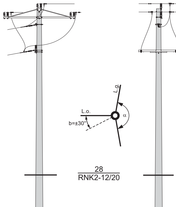
Słup rozgałęźny narożno - krańcowy RNK2 - □/□
