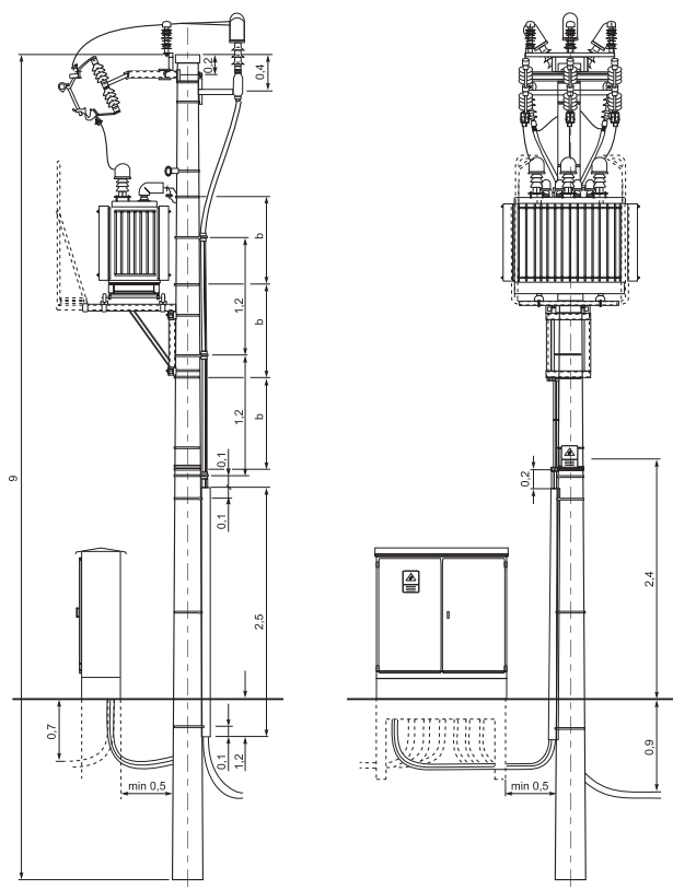
STSR - 20/400 - KK1
