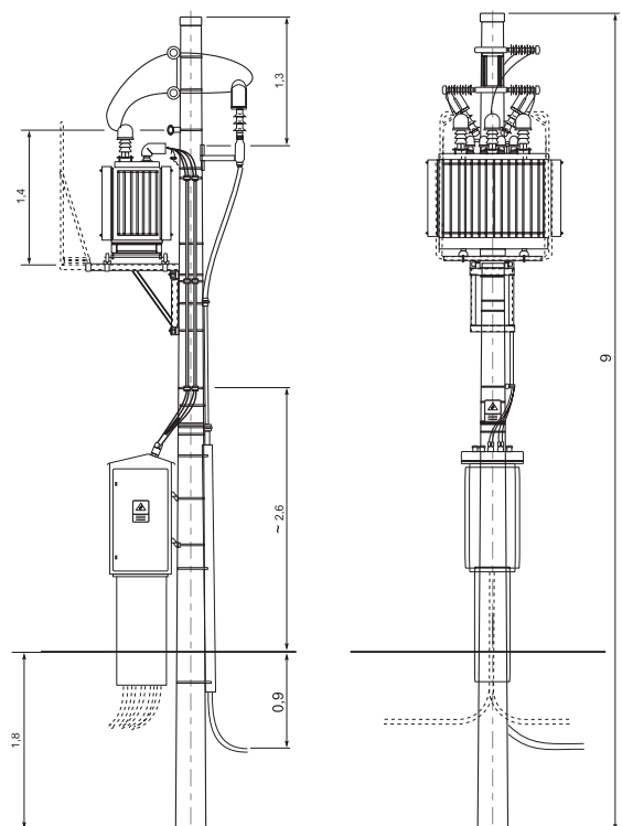
STSRu - 20/250 - KK1
