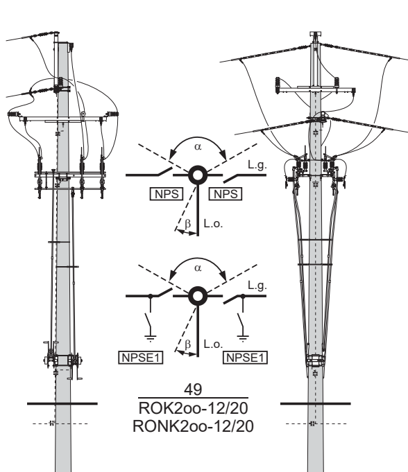
Słup rozgałęźny odporowo-krańcowy ROK2oo-□/□ i odporowo-narożno-krańcowy RONK2oo-□/□ z dwoma rozłącznikami NPS lub NPSE1
