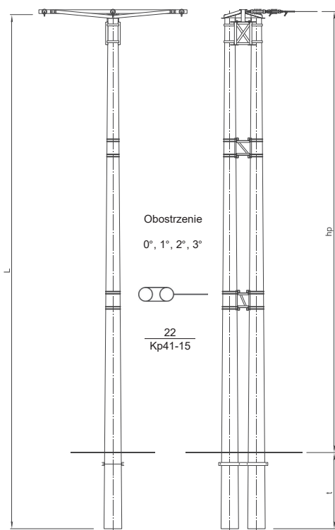
SŁUP KRAŃCOWY Kp41, Kp42
