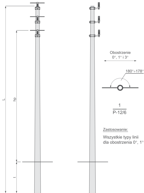
Słup przelotowy P - □/□□
