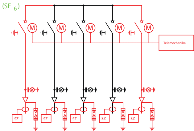
Front złącza
