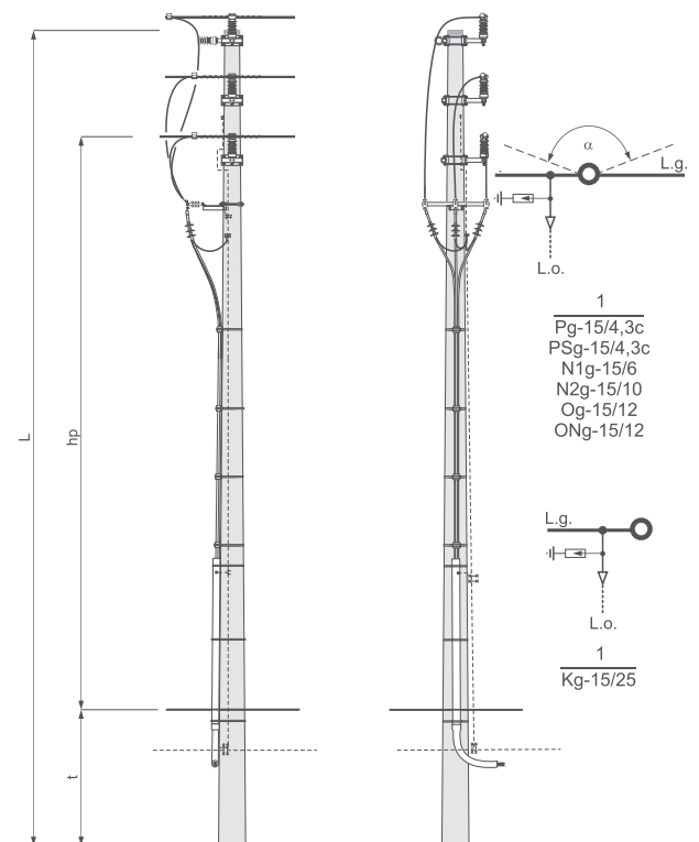
Słup przelotowy Pg-□/□□, skrzyżowaniowy PSg-□/□□, narożny N□g-□/□□ odporowy Og-□/□□, odporowo-narożny ONG-□/□□, krańcowy Kg-□/□□ z głowicami kablowymi
