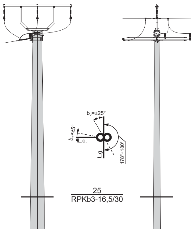
Słup rozgałęźny przelotowo - krańcowy bliźniaczy RPKb3 - □/□
