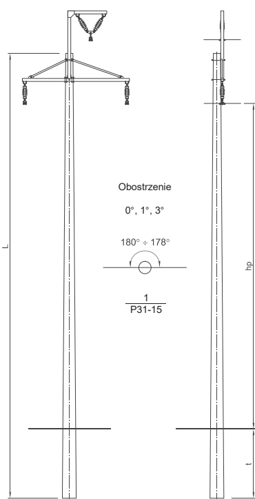
SŁUP PRZELOTOWY P31, P32
