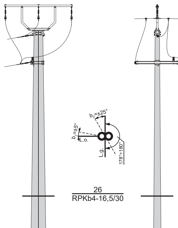
Słup rozgałęźny przelotowo - krańcowy bliźniaczy RPKb4 - □/□
