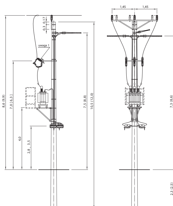
STNP-20/□/1
