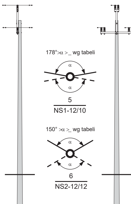
Słup narożno-skrzyżowaniowy NS1 - □/□□ dla \alpha \geq 150^\circ NS2 - □/□□ dla \alpha \geq 120^\circ
