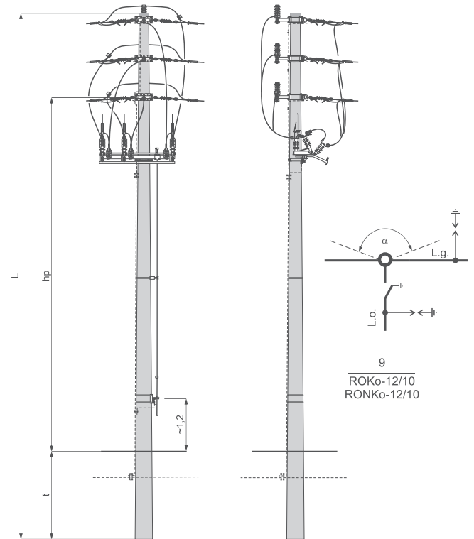
Słup rozgałęźny odporowo - krańcowy ROKo-□/□□ i rozgałęźny odporowo - krańcowy RONKo-□/□□ z rozłącznikiem FL□GBW-I lub FL□GBWu-I
