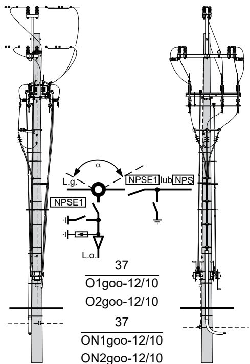
Słup odporowy O1goo, O2goo i odporowo-narożny ON1goo, ON2goo z głowicami kablowymi i rozłącznikiem NPSE1 oraz rozłącznikiem NPSE1 lub NPS
