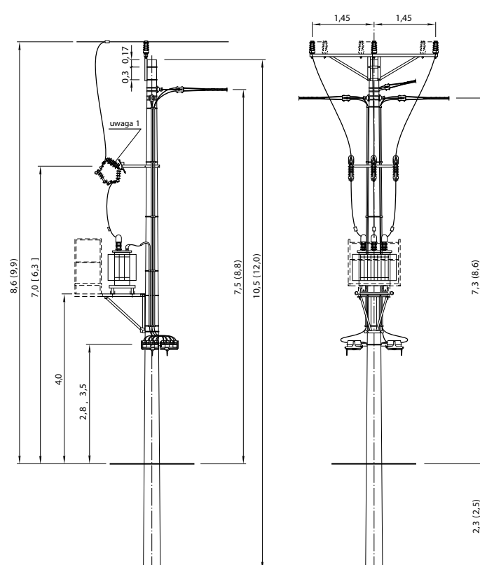
STNP-20/□/1
