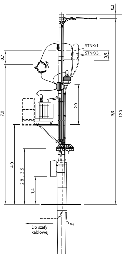
STNK-20/□/1/PP3, STNK-20/□/3/PP3
