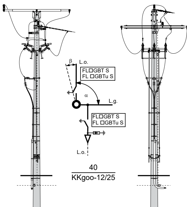
Słup odporowy KKgoo - □/□ z głowicami kablowymi i dwoma rozłącznikami FLGBT S lub FLGBTu S
