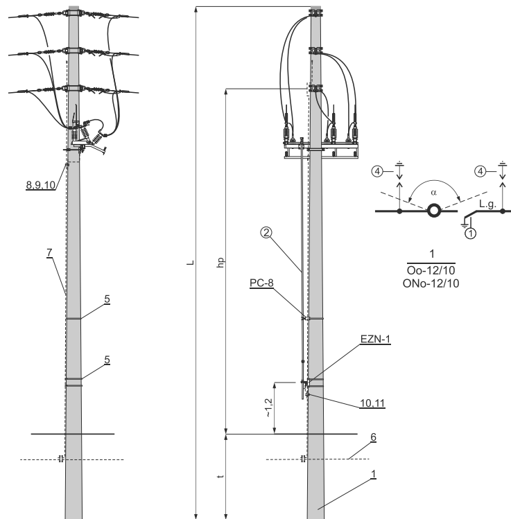
Słup odporowy Oo-□/□□ i odporowo-narożny ONo-□/□□ z rozłącznikiem FL□GB□-I lub FL□GB□u-I
