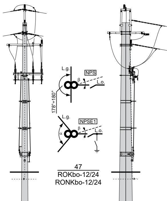
Słup rozgałęźny odporowo-krańcowy ROKbo-□/□ i odporowo-narożno-krańcowy RONKbo-□/□ - bliźniaczy z rozłącznikiem NPS lub NPSE1
