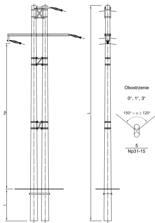
SŁUP NAROŻNY Np31, Np32 dla 150^\circ > \alpha \geq 120^\circ
