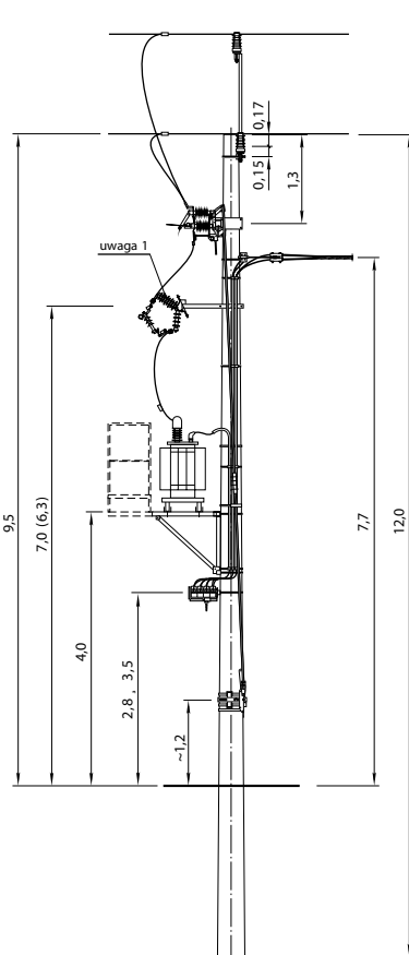
STNP-20/□/2
