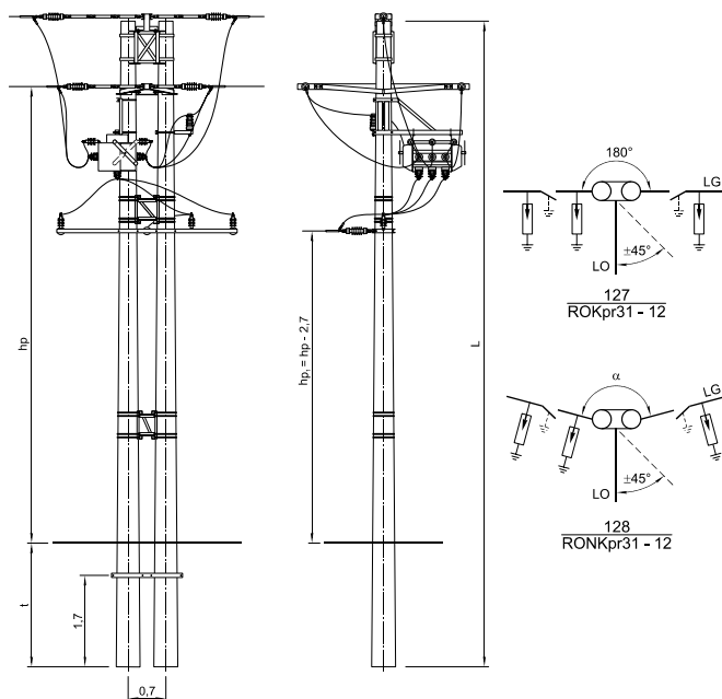
SŁUP ROZGAŁĘŻNY ODPOROWO-KRAŃCOWY ROKpr31÷ROKpr33 i ODPOROWO-NAROŻNO-KRAŃCOWY RONKpr31÷RONKpr33 Z ROZŁĄCZNIKIEM SECTOS NXBD
