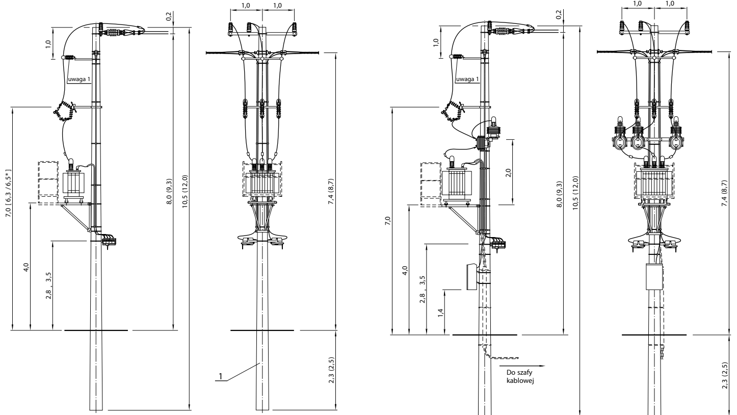
STN-20 /□/II
