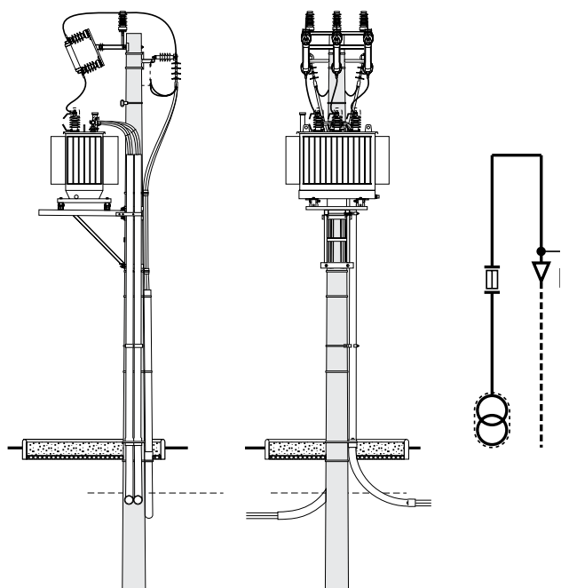
STSRS - 20/630-KK1-8,2/10 kablowa krótka
