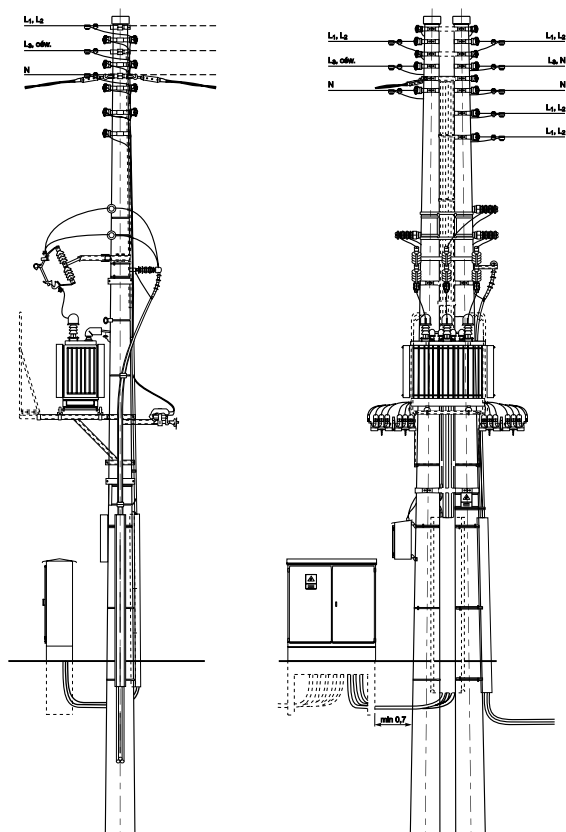
STSRp - 20/400 - K2
