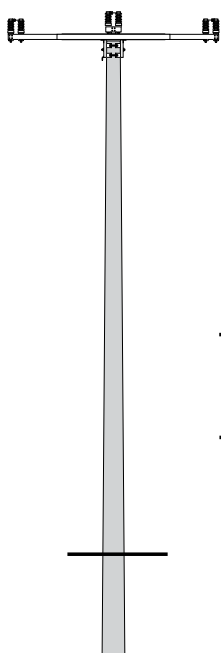
Słup przelotowo - skrzyżowaniowy PS1 - □/10□ i narożno - skrzyżowaniowy NS1-□/□□
