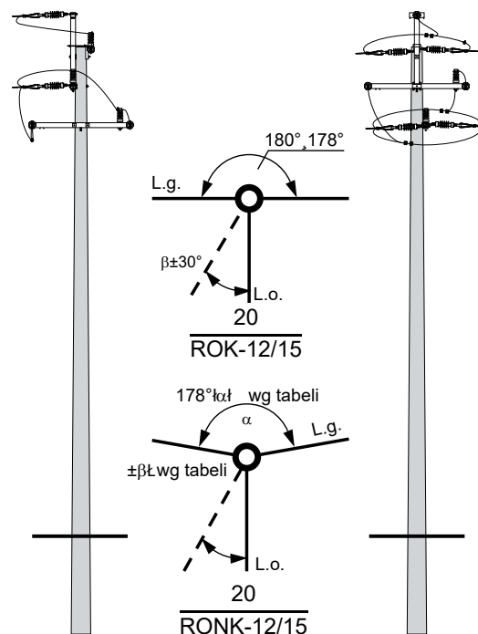
Słup rozgałęźny odporowo - krańcowy ROK - □/□□ i odporowo - narożno - krańcowy RONK - □/□□
