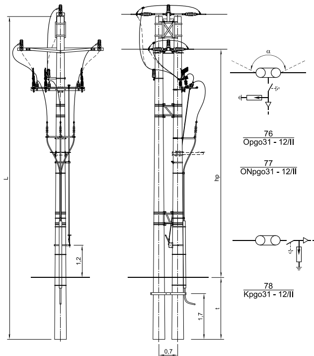
SŁUP ODPOROWY Opgo31, ODPOROWO-NAROŻNY ONpgo31÷ONpgo33 i KRAŃCOWY Kpgo31, Kpgo32 Z GŁOWICAMI KABLOWYMI I ODŁĄCZNIKIEM SON, SOUN LUB ROZŁĄCZNIKIEM SRN, SRUN WARIANT II
