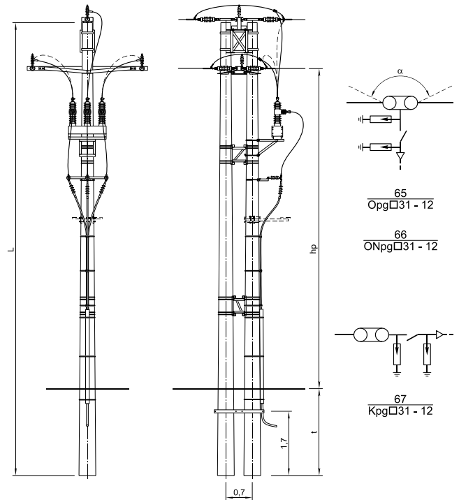
SŁUP ODPOROWY Opg□31, ODPOROWO-NAROŻNY ONpg□31÷ONpg□33 i KRAŃCOWY Kpg□31, Kpg□32 Z ROZŁĄCZNIKIEM DAS LUB WYŁĄCZNIKIEM GVR
