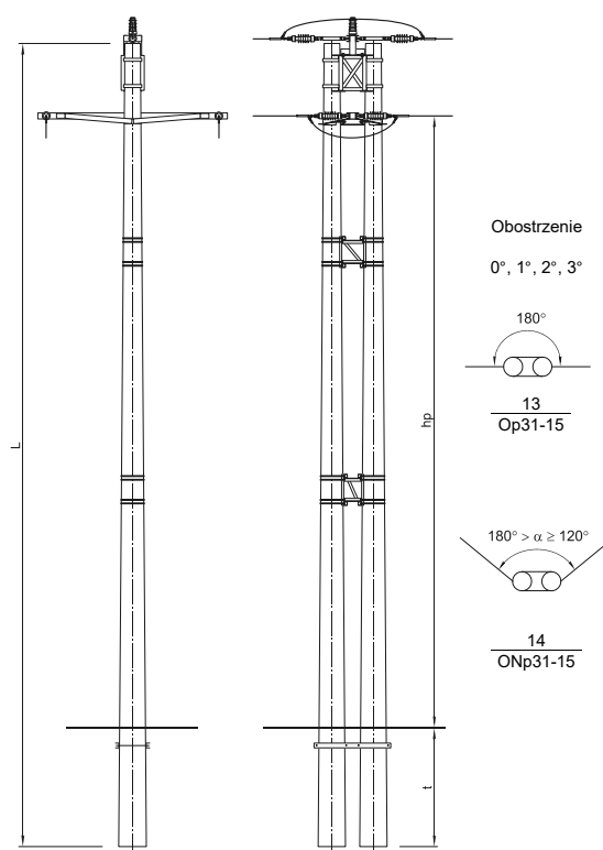
SŁUP ODPOROWY Op31 I ODPOROWO-NAROŻNY ONp31, ONp32, ONp33
