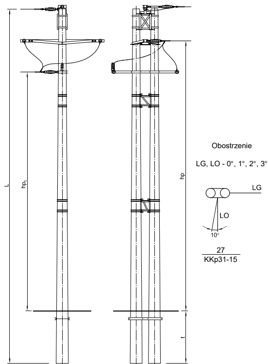
SŁUP KRAŃCOWO-KRAŃCOWY KKp31, KKp32, KKp33
