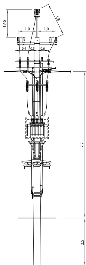
STNKso-20/□/II, STNKpo-20/□/II
