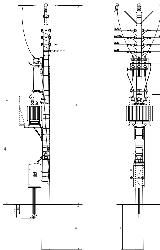
STSRu - 20/250 - p
