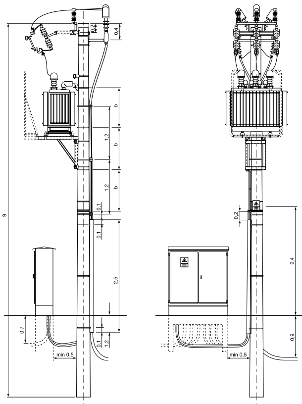
STSR - 20/400 - KK1
