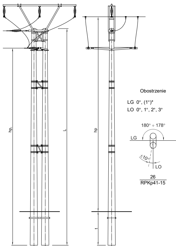
SŁUP ROZGAŁĘŻNY PRZELOTOWO-KRAŃCOWY RPKp41, RPKp42, RPKp43
