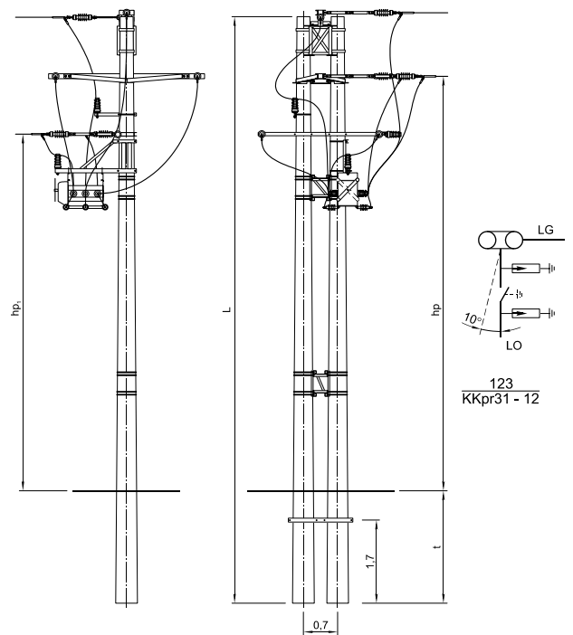
SŁUP KRAŃCOWO-KRAŃCOWY KKpr31÷KKpr33 Z ROZŁĄCZNIKIEM SECTOS NXB
