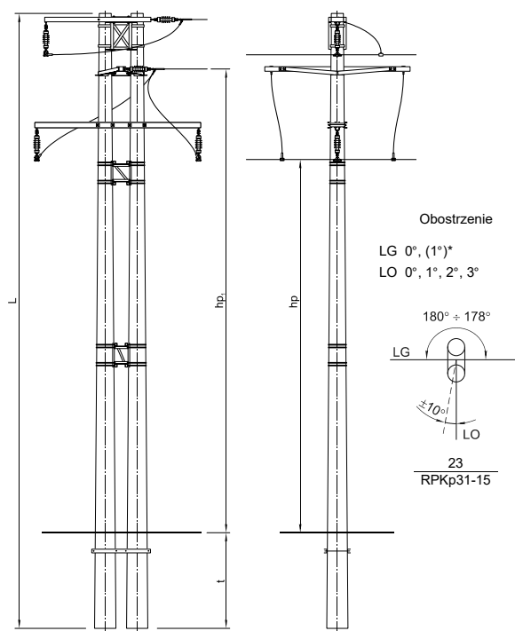
SŁUP ROZGAŁĘŻNY PRZELOTOWO-KRAŃCOWY RPKp31, RPKp32, RPKp33
