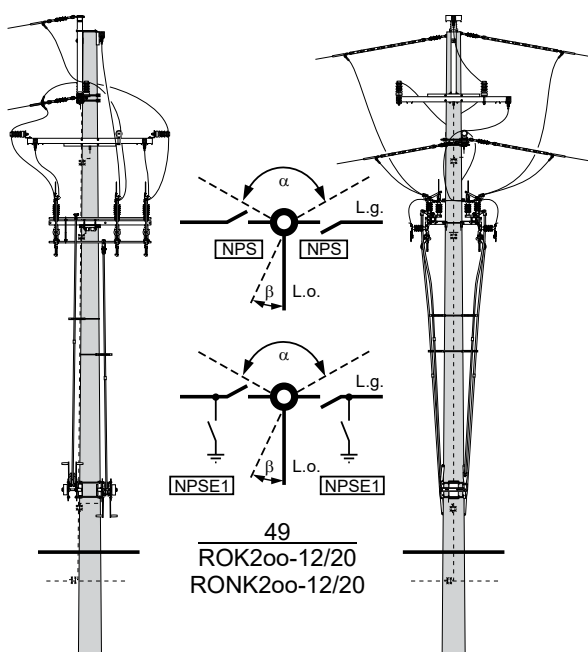
Słup rozgałęźny odporowo-krańcowy ROK2oo-□/□ i odporowo-narożno- krańcowy RONK2oo-□/□ z dwoma rozłącznikami NPS lub NPSE1
