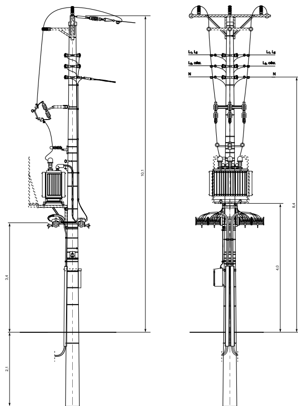
STSR - 20/400 - Wariant I
