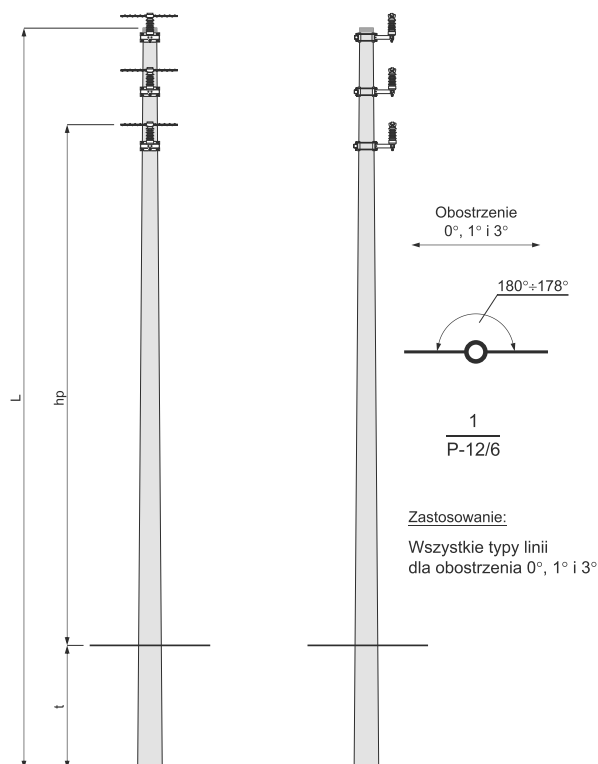
Słup przelotowy P - □/□□
