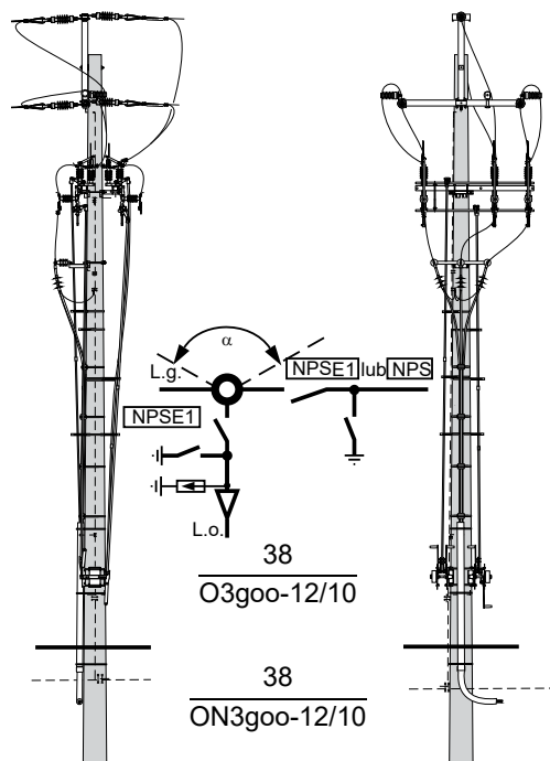
Słup odporowy O3goo-□/□□ i odporowo-narożny- ON3goo-□/□□ z głowicami kablowymi i rozłącznikiem NPSE1 oraz rozłącznikiem NPSE1 lub NPS
