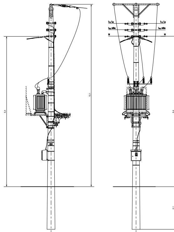
STSRu - 20/250 - Wariant IA
