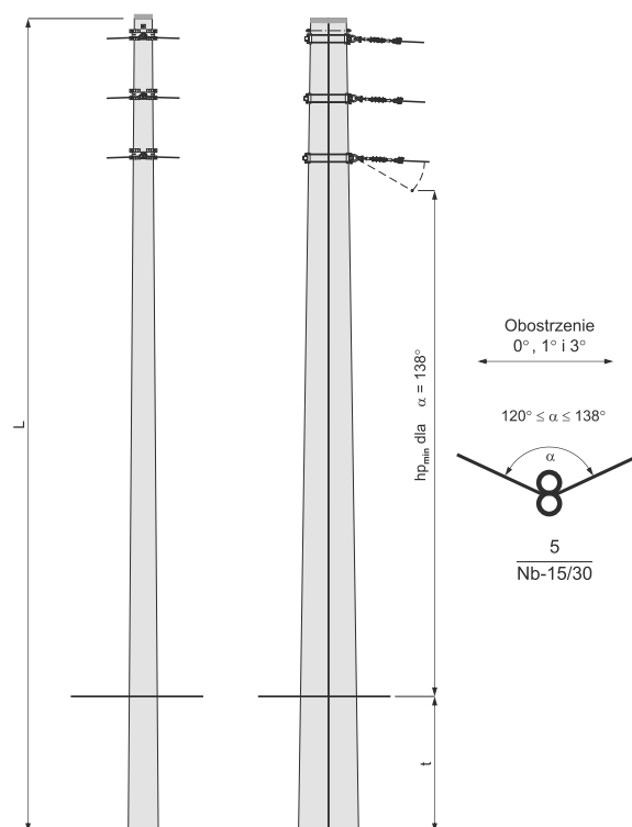
Słup narożny bliźniaczy Nb - □/□
