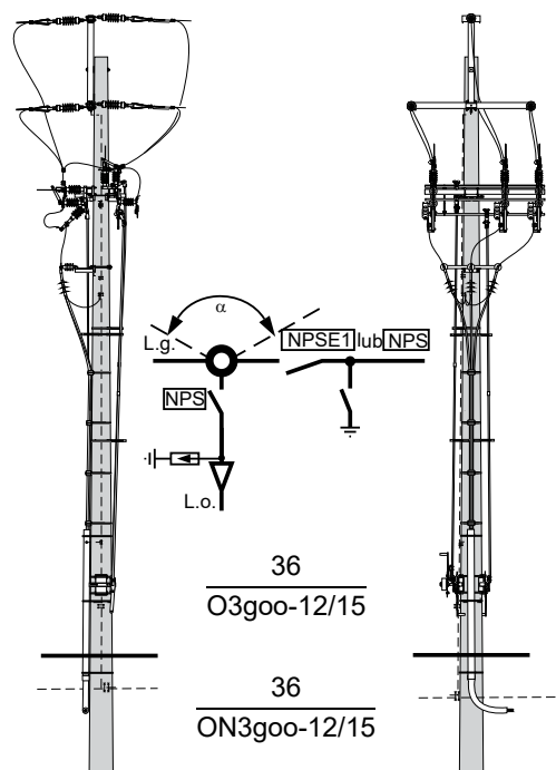
Słup odporowy O3goo i odporowo-narożny ON3goo z głowicami kablowymi i rozłącznikiem NPS oraz rozłącznikiem NPSE1 lub NPS
