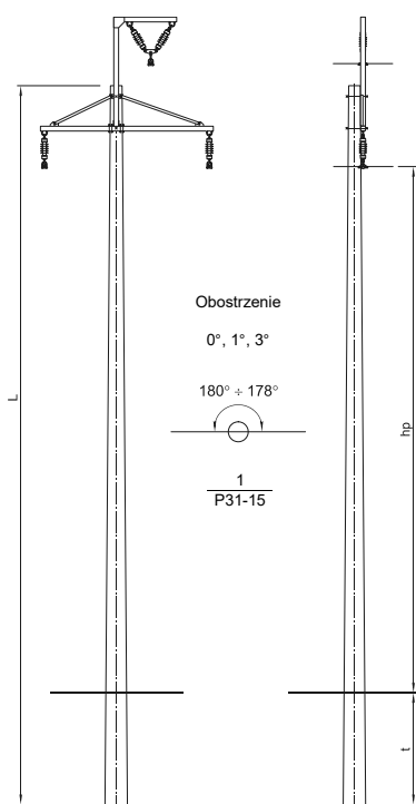
SŁUP PRZELOTOWY P31, P32
