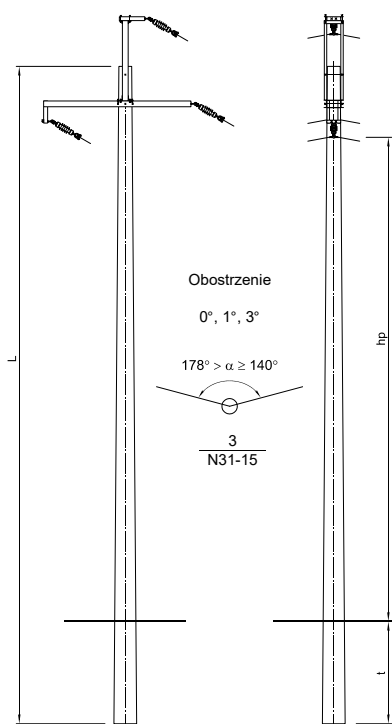
SŁUP NAROŻNY N31, N32, N33, N34, N35 i N36 dla 178^\circ > \alpha \geq 140^\circ
