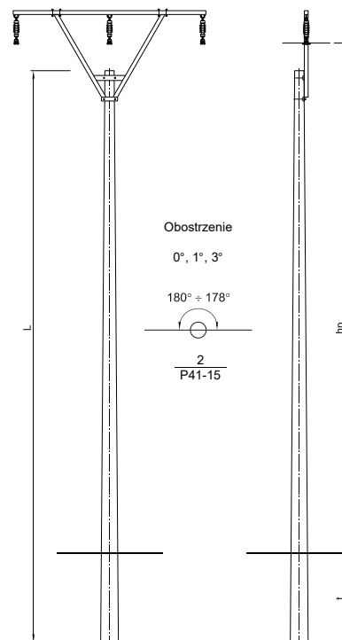
SŁUP PRZELOTOWY P41, P42
