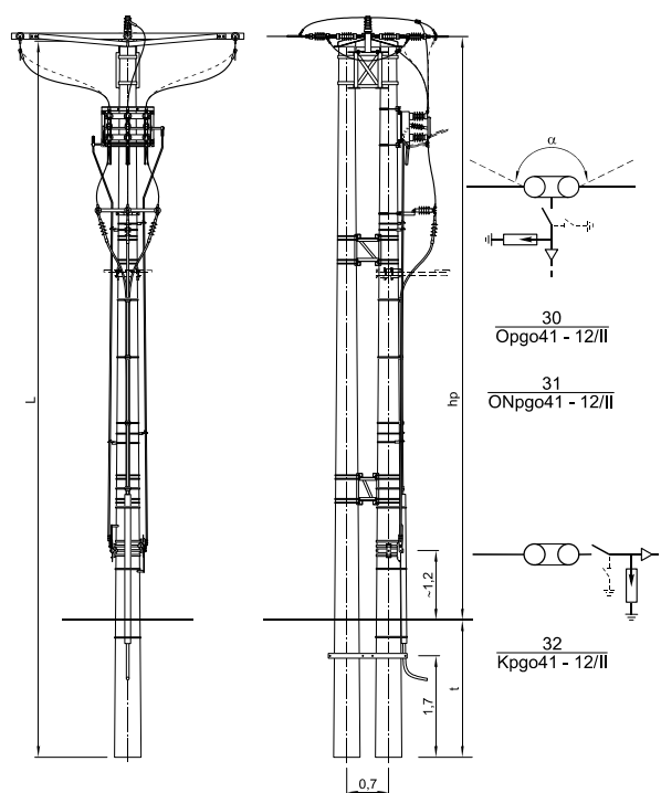
SŁUP ODPOROWY Opgo41, ODPOROWO-NAROŻNY ONpgo41÷ONpgo43 i KRAŃCOWY Kpgo41, Kpgo42 Z GŁOWICAMI KABLOWYMI I ODŁĄCZNIKIEM ON III
