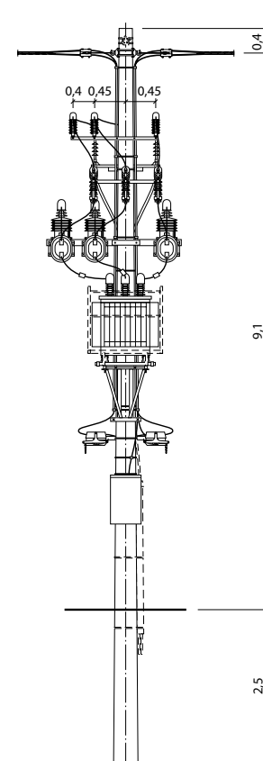
STNK-20/□/1/PP3, STNK-20/□/3/PP3
