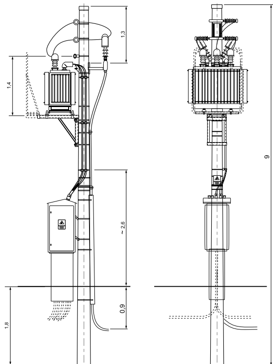
STSRu - 20/250 - KK1
