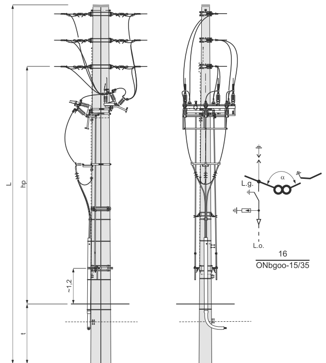
Słup odporowo-narożny ONbgoo-□/□ bliźniaczy z głowicami kablowymi i rozłącz. FL□GBT S lub FL□GBTu S oraz rozłącz. FL□GB□-I lub FL□GB□u-I
