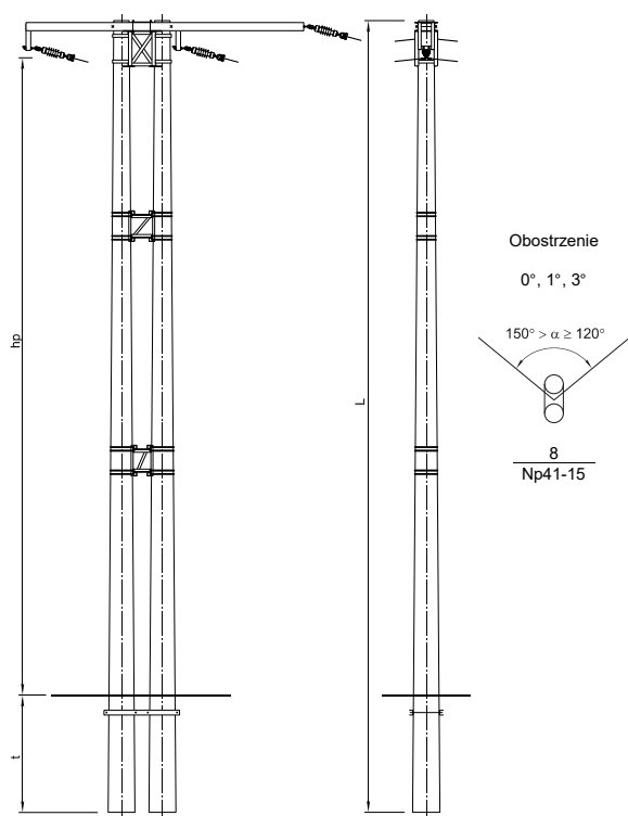
SŁUP NAROŻNY Np41, Np42 dla 150^\circ > \alpha \geq 120^\circ
