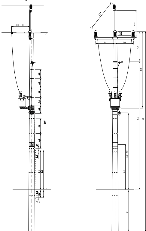
STSR - P0 - 20/25 - I - p
