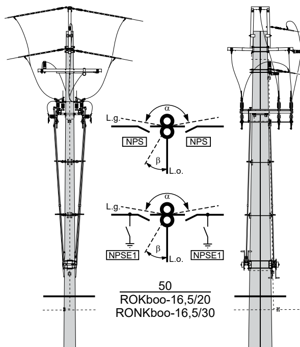
Słup rozgałęźny odporowo-krańcowy ROKboo-□/□ i odporowo-narożno- krańcowy RONKboo-□/□ - bliźniaczy z dwoma rozłącznikami NPS lub NPSE1
