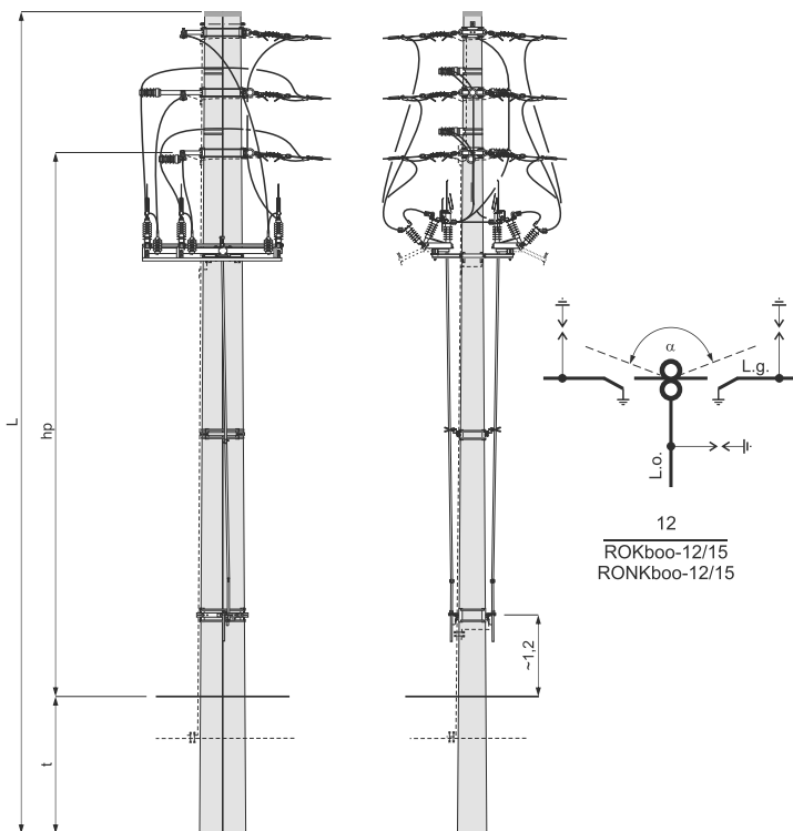
Słup rozgałęźny odporowo - krańcowy bliźniaczy ROK12-□/□ i rozg. odp. - narożno krańcowy bliźniaczy RONK12-□/□ z rozłącznikiem FLGBW-I lub FLGBWu-I i rozłącznikiem FLGBWL-I lub FLGBWLu-I
