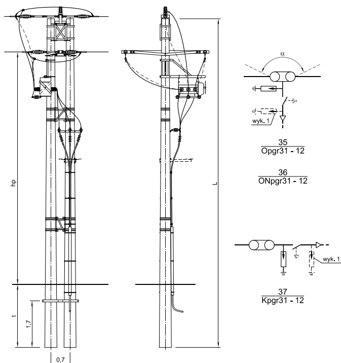
SŁUP ODPOROWY Opgr31, ODPOROWO-NAROŻNY ONpgr31÷ONpgr33 i KRAŃCOWY Kpgr31, Kpgr32 Z GŁOWICAMI KABLOWYMI I ROZŁĄCZNIKIEM SECTOS NXB
