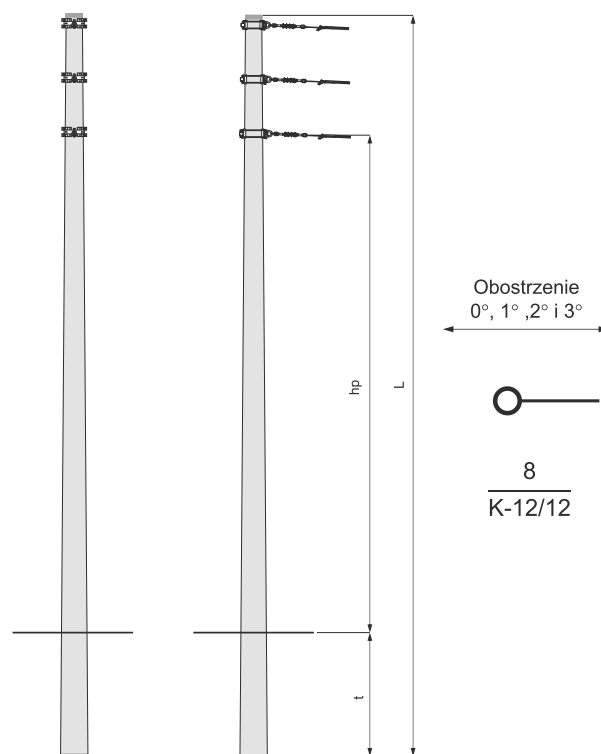
Słup krańcowy K - □/□□
