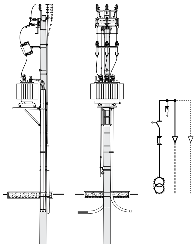
STSRS - 20/630-K-10,5/10-0 z odłącznikiem
