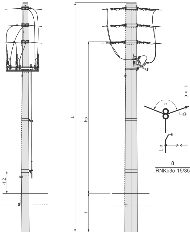
Słup rozgałęźny narożno - krańcowy bliźniaczy RNB30-□/□ z rozłącznikiem FLGBW-I lub FLGBWu-I
