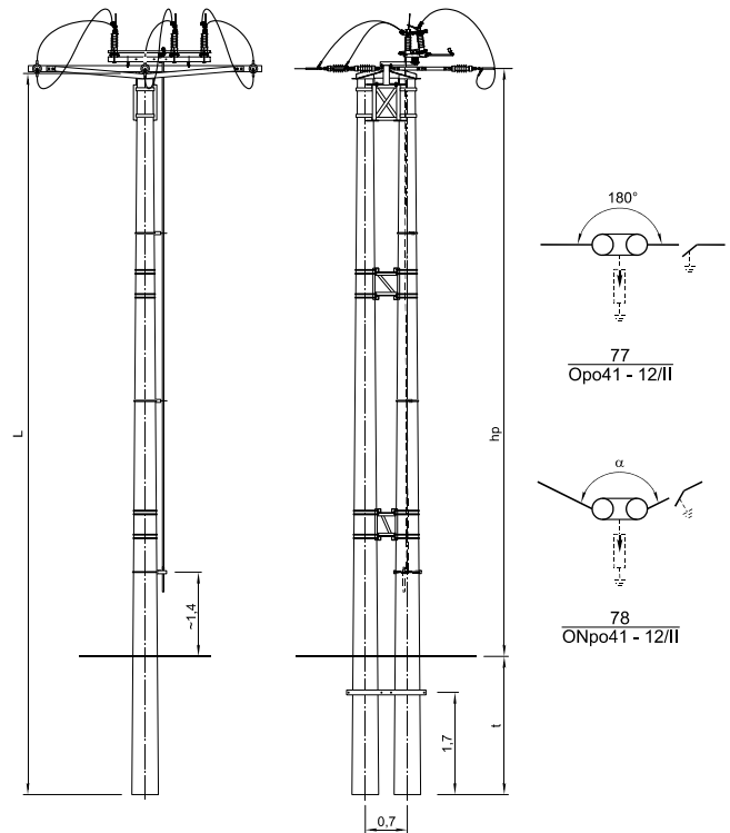
SŁUPA ODPOROWY Opo41 i ODPOROWO-NAROŻNY ONpo41÷ONpo43 Z ODŁĄCZNIKIEM ON M III SA, OUN M III SA LUB ROZŁĄCZNIKIEM RN M III SA, RUN M III SA WARIANT I
