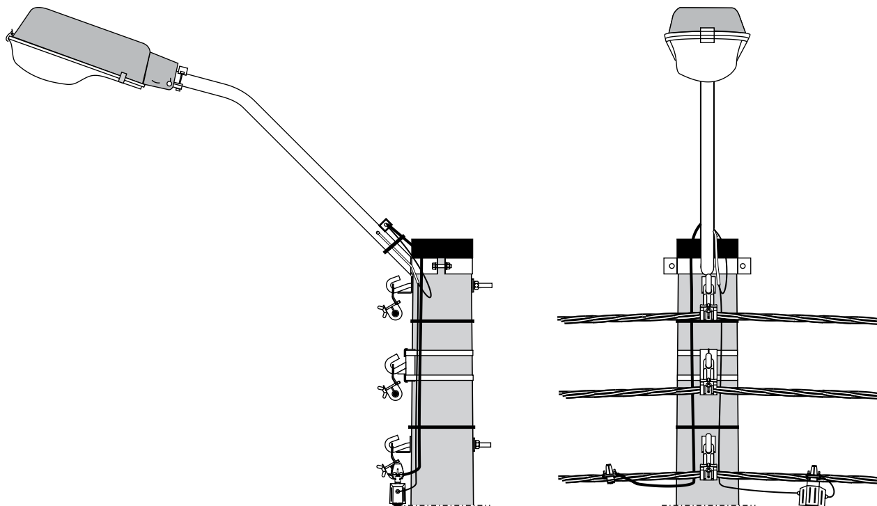
A. Oprawa nad przewodami linii
