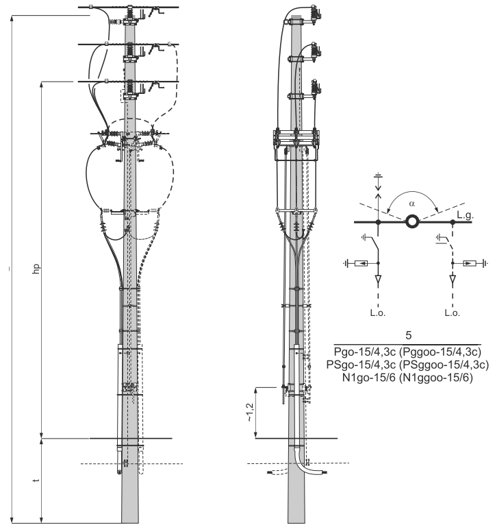
Słup przelotowy Pgo - □/□□, skrzyżowaniowy PSgo - □/□□, narożny N1go-□/□□ z głowicami kablowymi i odłącznikiem ONp, OUNp lub rozłącznikiem RNp, RUNp
