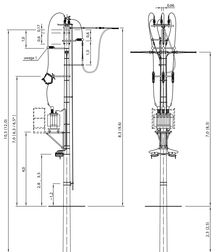
STNKso-20/□/II, STNKpo-20/□/II
