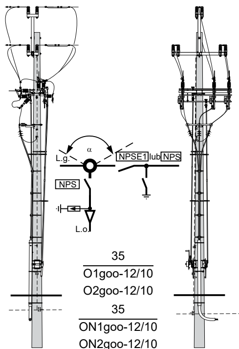
Słup odporowy O1goo, O2goo i odporowo-narożny ON1goo, ON2goo z głowicami kablowymi i rozłącznikiem NPS oraz rozłącznikiem NPSE1 lub NPS
