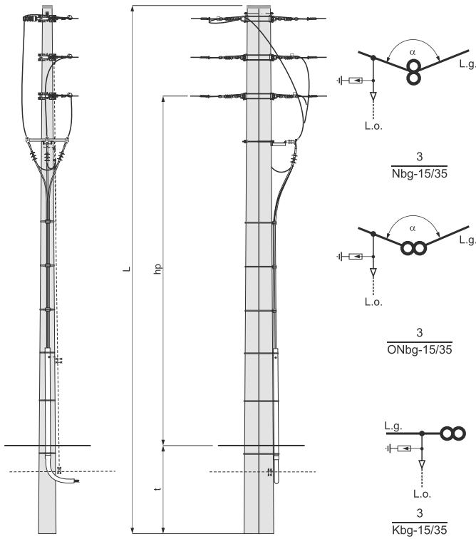
Słupy narożny Nbg-□/□ odporowo-narożny ONbg- □/□, krańcowy Kg - □/35 - bliźniaczy z głowicami kablowymi
