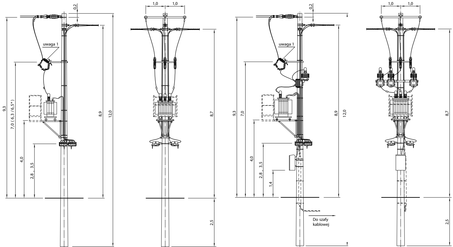
STN-20 /□/I
