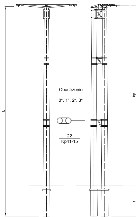
SŁUP KRAŃCOWY Kp41, Kp42
