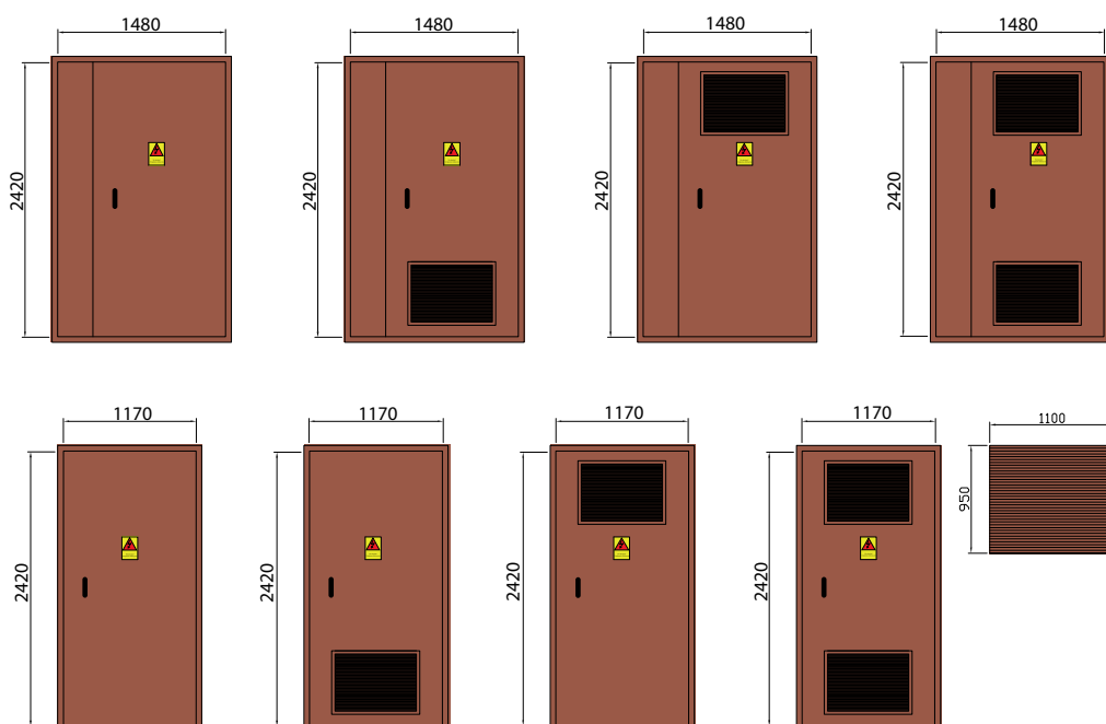
Zastosowanie w stacjach KSW 296/... o wysokořci korpusu 2970 mm
