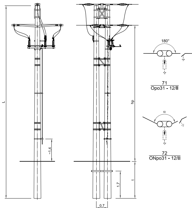
SŁUPA ODPOROWY Opo31 i ODPOROWO-NAROŻNY ONpo31÷ONpo33 Z ODŁĄCZNIKIEM ON M III SA, OUN M III SA LUB ROZŁĄCZNIKIEM RN M III SA, RUN M III SA WARIANT II
