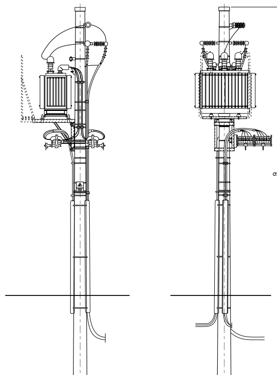
STSRu - 20/250 - KK2
