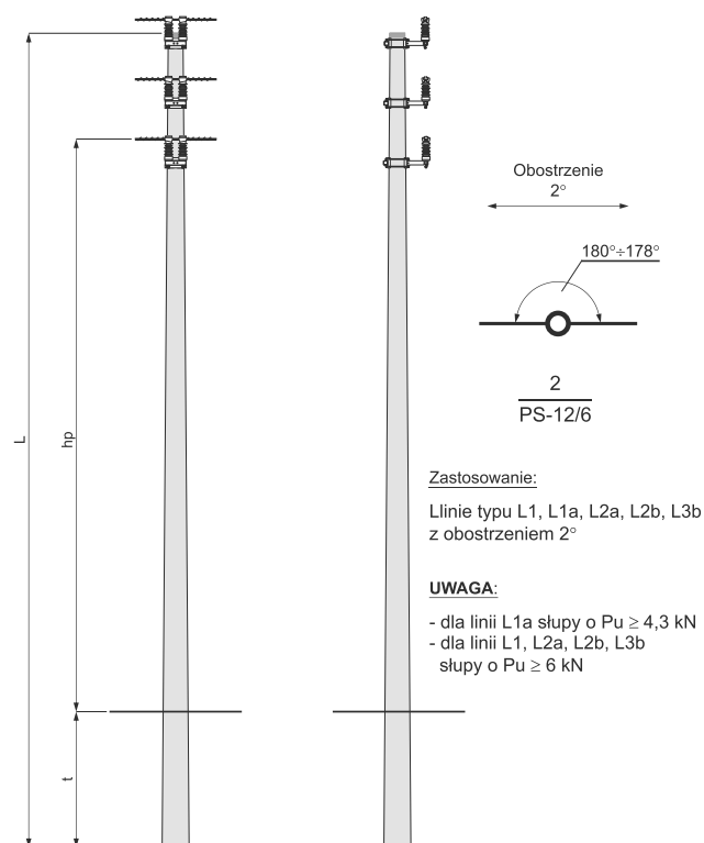
Słup przelotowo-skrzyżowaniowy PS - □/□□
