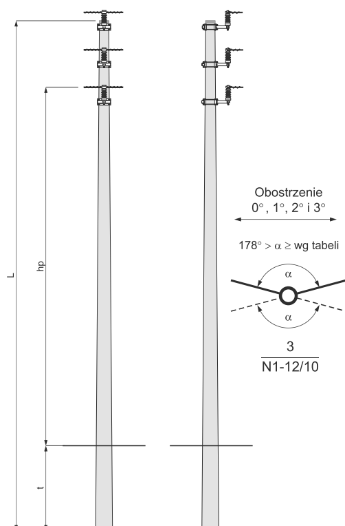
Słup narożny N1 - □/□□ \alpha \geq 150^\circ
