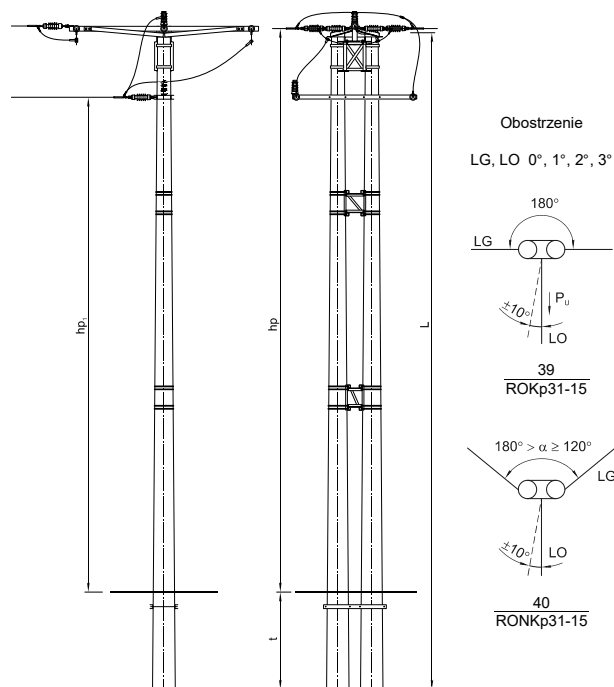
SŁUP ROZGAŁĘŻNY ODPOROWO-KRAŃCOWY ROKp41+ROKp43 i ODPOROWO-NAROŻNO-KRAŃCOWY RONKp41+RONKp43
