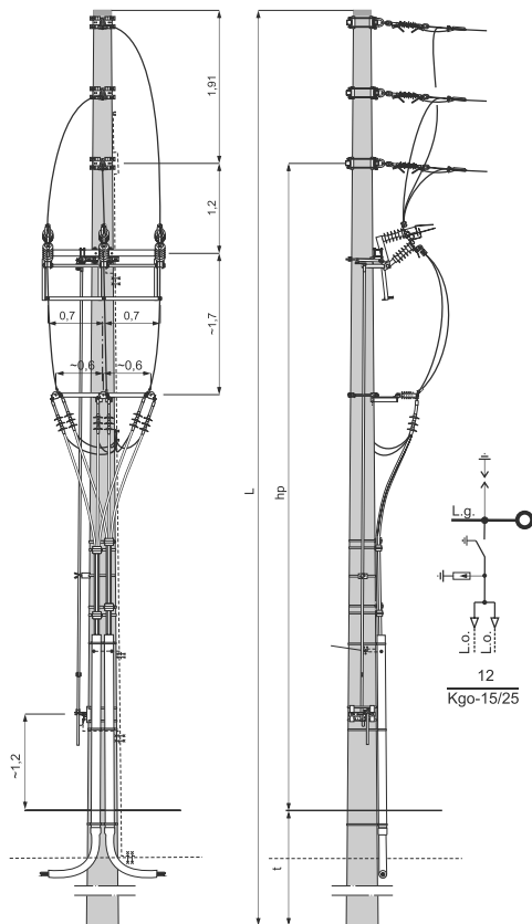
Słup krańcowy Kggoo - □/□□ z dwoma kompletami głowic kablowych i rozłącznikiem FL□GBT S lub FL□GBTu S
