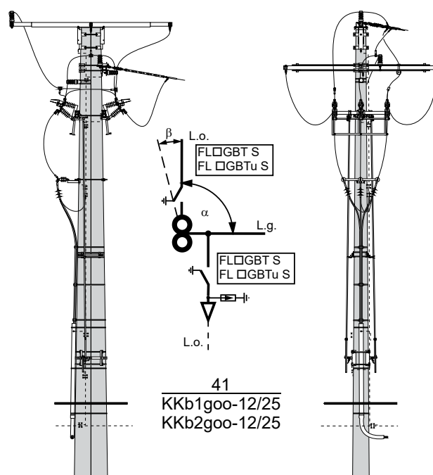
Słup krańcowo - krańcowy KKb1goo - □/□, KKb2goo - □/□ - bliźniaczy z głowicami kablowymi i dwoma rozłącznikami FLGBT S lub FLGBTu S
