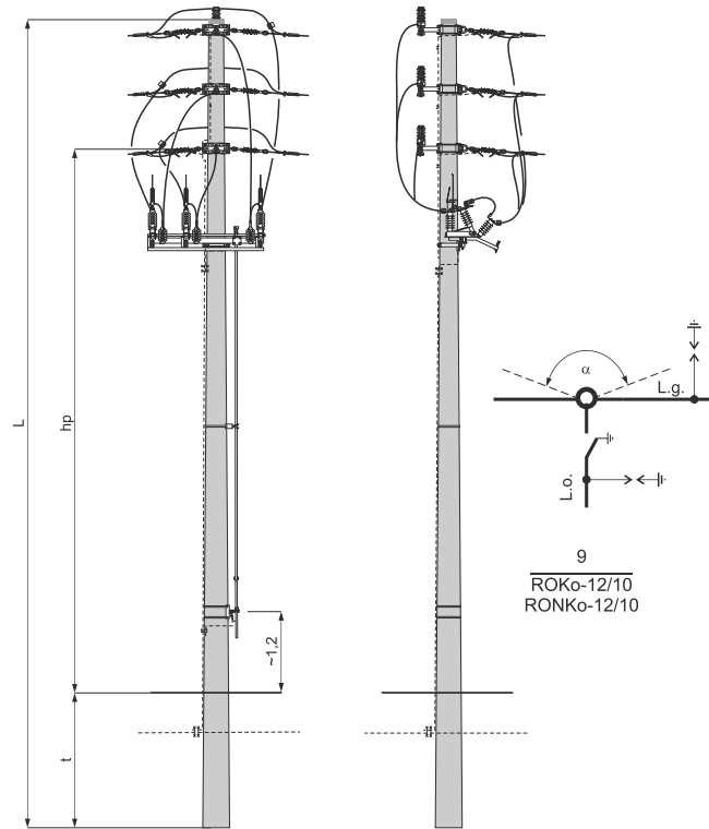
Słup rozgałęźny odporowo - krańcowy ROK12-□/□ i rozgałęźny odporowo - krańcowy RONK12-□/□ z rozłącznikiem FLGBW-I lub FLGBWu-I
