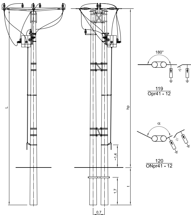
SŁUP ODPOROWY Opr41 i ODPOROWO-NAROŻNY ONpr41÷ONpr43 Z ROZŁĄCZNIKIEM THO
