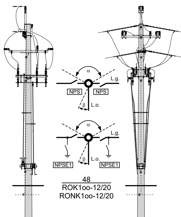
Słup rozgałęźny odporowo-krańcowy ROK1oo-□/□ i odporowo-narożno- krańcowy RONK1oo-□/□ z dwoma rozłącznikami NPS lub NPSE1
