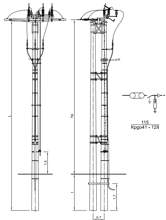
SŁUP KRAŃCOWY Kpgo41, Kpgo42 Z GŁOWICAMI KABLOWYMI I ODŁĄCZNIKIEM ON III-W, OUN III-W, ON M, OUN M LUB ROZŁĄCZNIKIEM RN III-W, RUN III-W, RN M, RUN M WARIANT I
