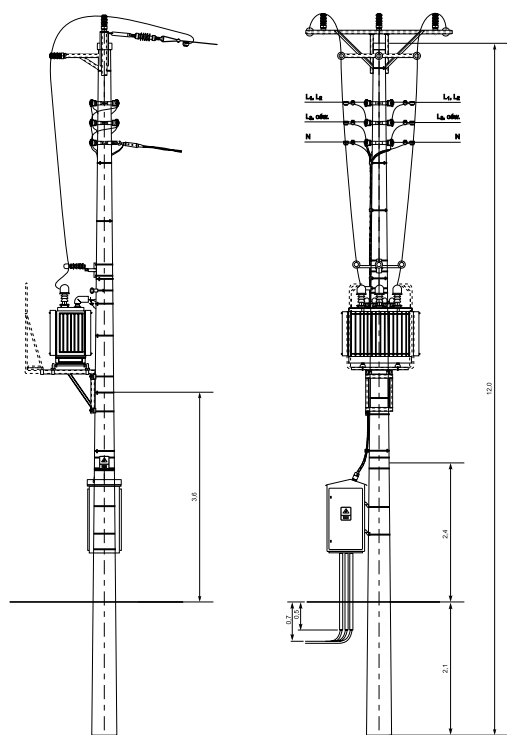
STSRu - 20/250 - Wariant I
