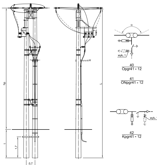
SŁUP ODPOROWY Opgr41, ODPOROWO-NAROŻNY ONpgr41÷ONpgr43 i KRAŃCOWY Kpgr41, Kpgr42 Z GŁOWICAMI KABLOWYMI I ROZŁĄCZNIKIEM SECTOS NXB
