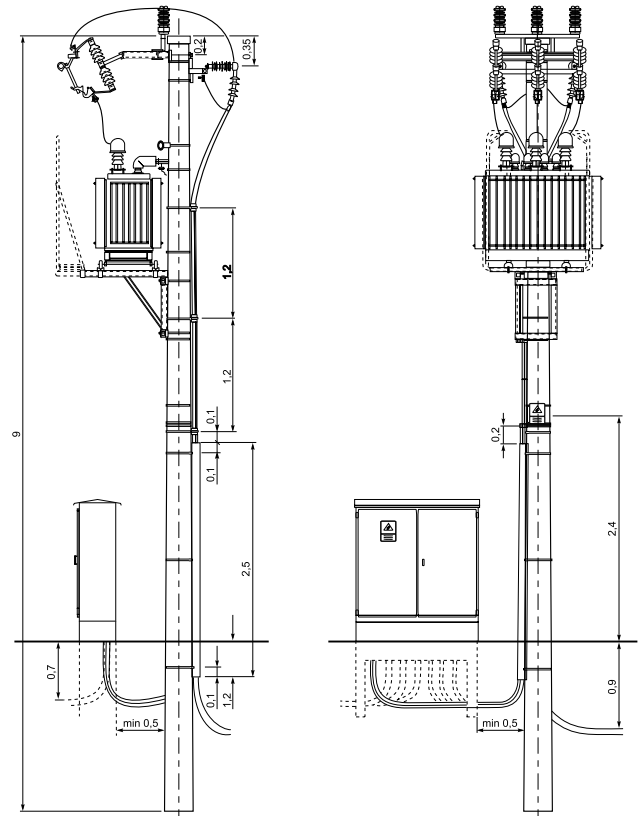
STSR - 20/400 - KK2
