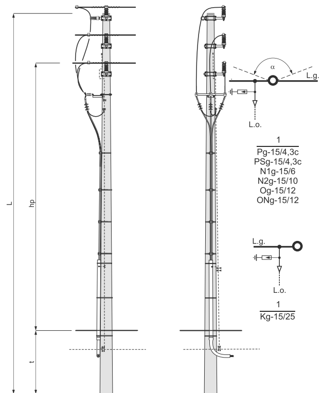
Słup przelotowy Pg15-□/□, skrzyżowaniowy PSg15-□/□, narożny N1g15-□/□ odporowy Og15-□/□, odporowo-narożny ONg15-□/□, krańcowy Kg15-□/□ z głowicami kablowymi
