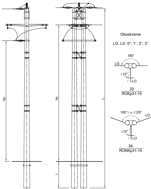
SŁUP ROZGAŁĘŻNY ODPOROWO-KRAŃCOWY ROKp31+ROKp33 i ODPOROWO-NAROŻNO-KRAŃCOWY RONKp31+RONKp33
